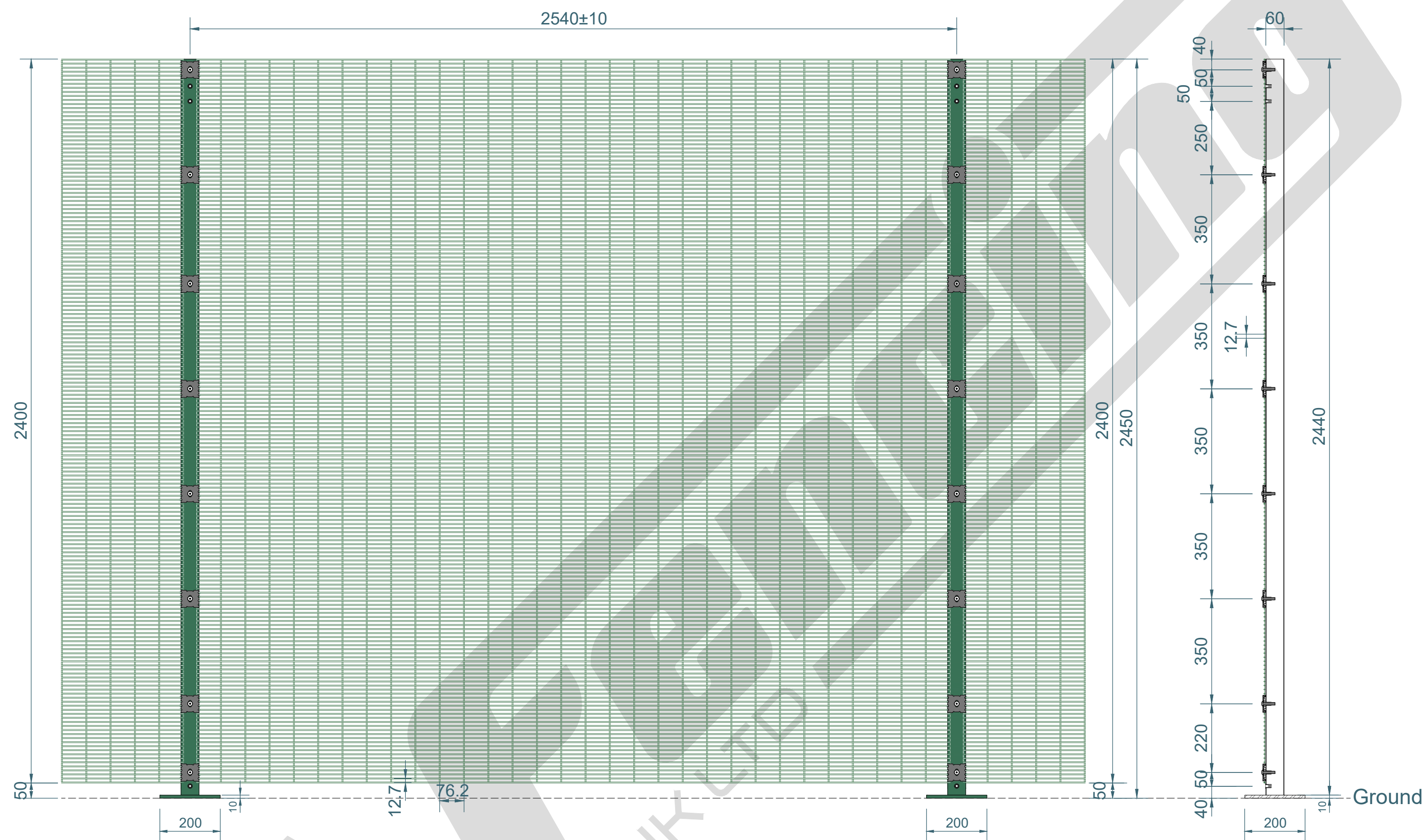
Elevation 1:12
