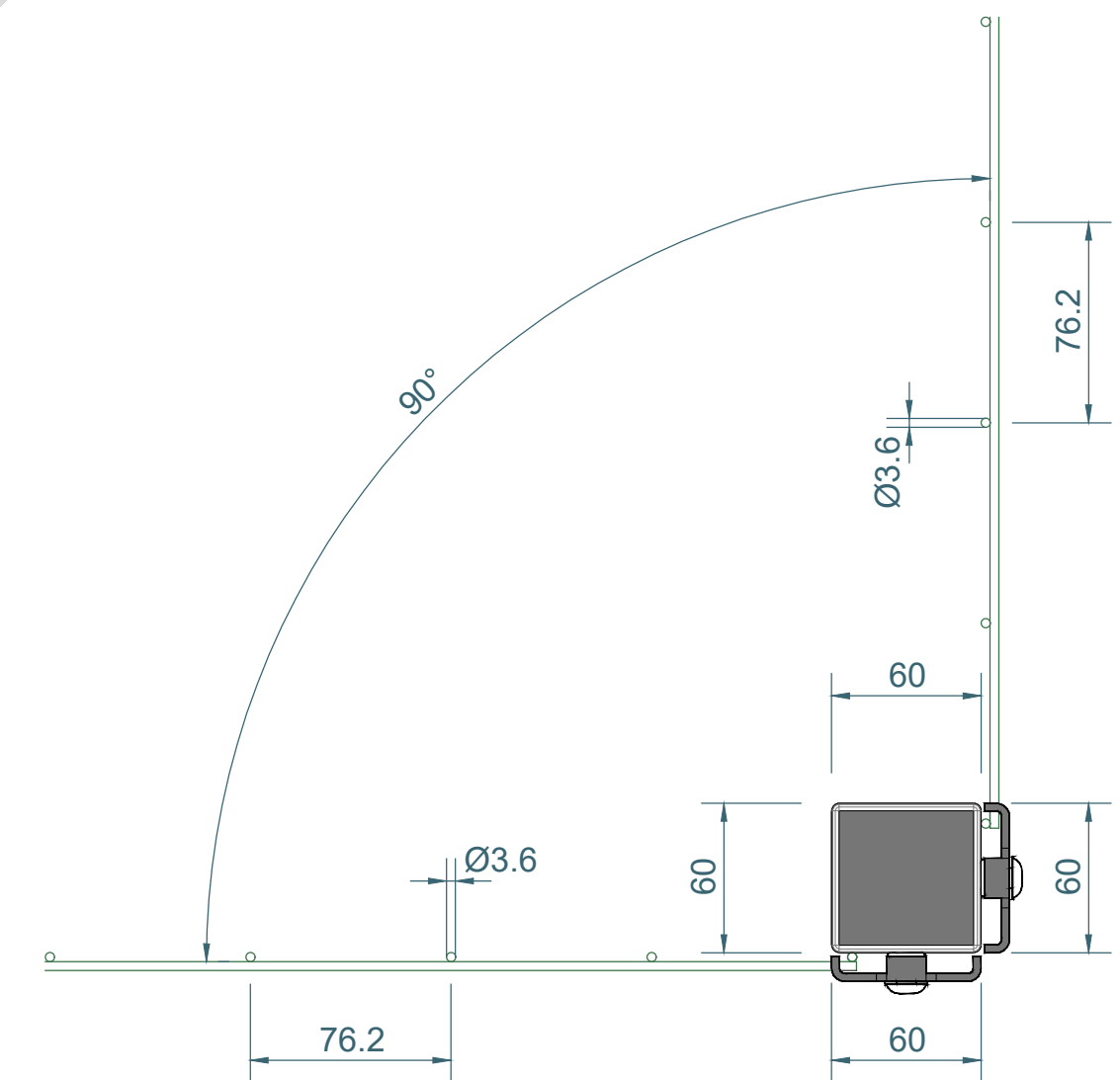
Top Plan 1:3
